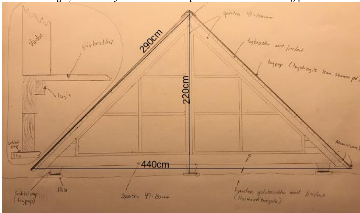
Fra ansøgningsmaterialet: facadetegning af shelter
